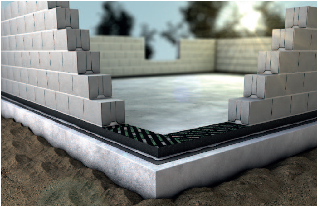
Mauerfußdämmung aus Schaumglas: – FOAMGLAS® PERINSUL HL
