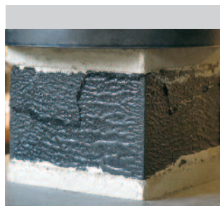
Bild 1: Zentrische Druckbelastung auf einen FOAMGLAS® PERINSUL Probekörper im Mörtelbett (Mörtel oben und unten).
