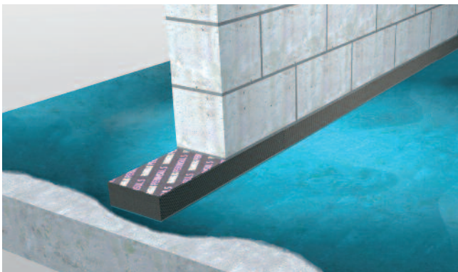
Mit PERINSUL
