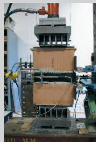
Bild 7: Scherversuch.
