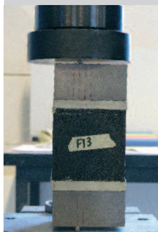
Bild 2: Exzentrische Druckbelastung auf einen FOAMGLAS® PERINSUL Prüfkörper.
