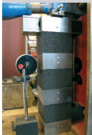
Bild 4: Kriechversuch mit FOAMGLAS® PERINSUL Prüfwürfeln.
